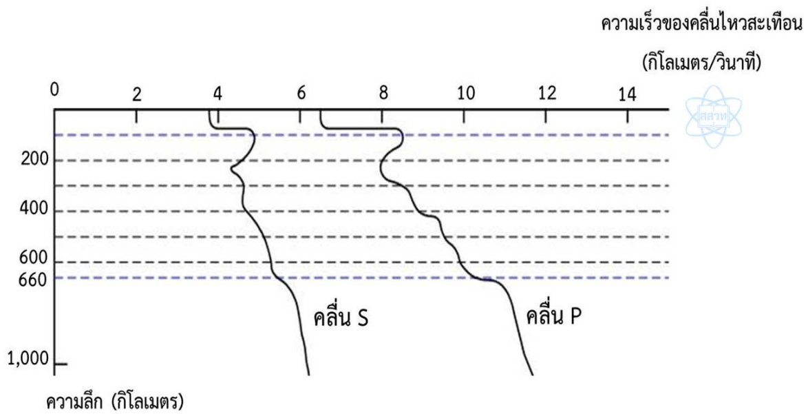
รูป 2 ภาพขยายกราฟแสดงความสัมพันธ์ระหว่างความเร็วของคลื่นไหวสะเทือน กับระดับความลึกช่วง 0-1,000 กิโลเมตร จากผิวโลก
